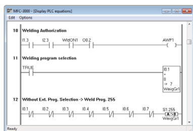
UKÁŽKA PLC PROGRAMU
